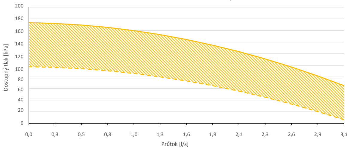
i-HPV5 0250 – PSI Provozní oblast čerpadla
