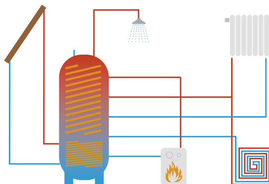
Schéma zapojení hygienického zásobníku ENBRA Caddy
