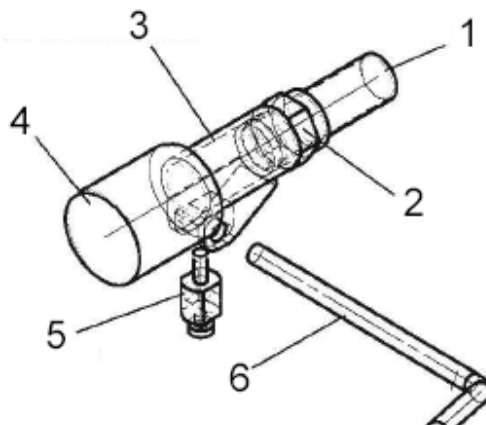
obr. 4: Termomechanický regulátor výkonu
